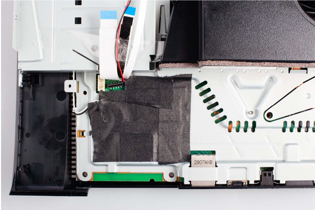
Illustration 11: Isolation de la plaque métallique
