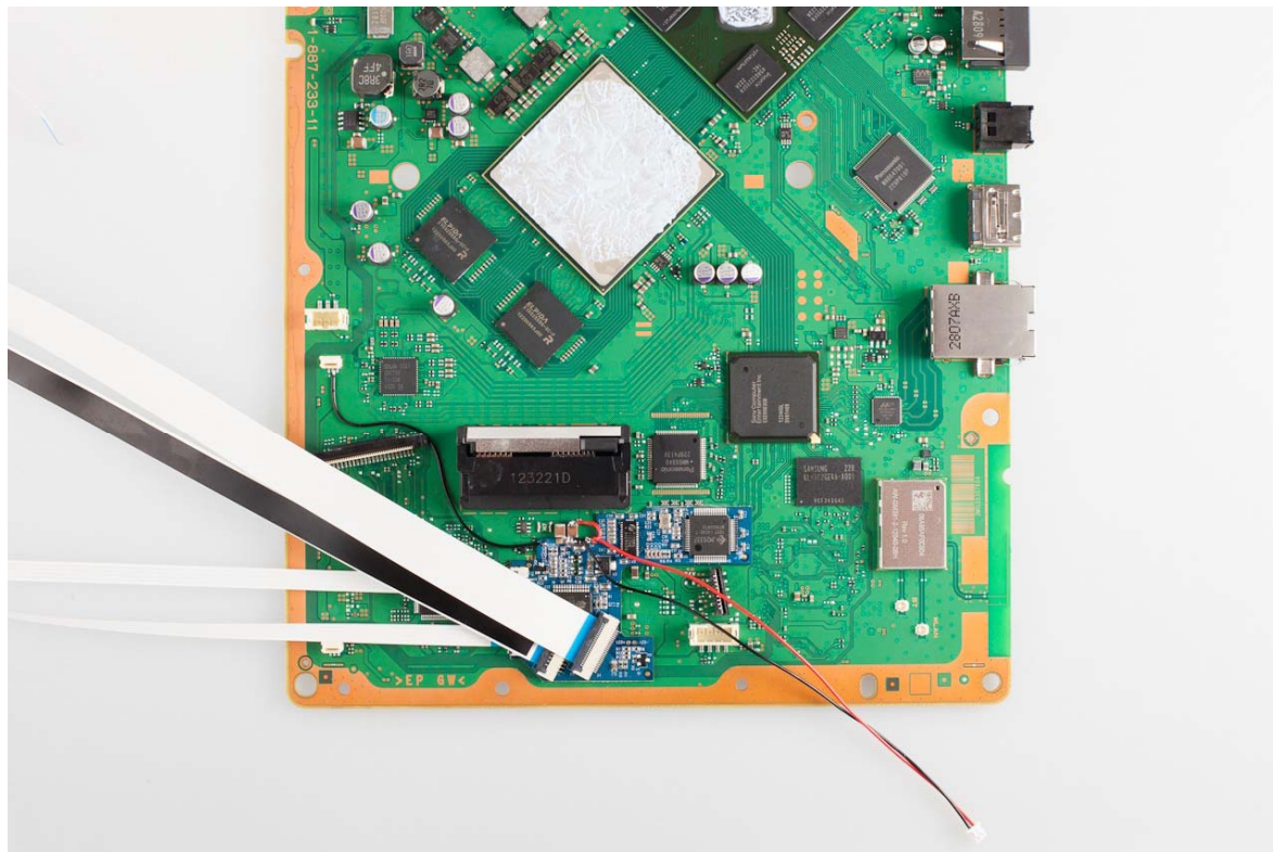
Illustration 7: positionnement des nappes souples
