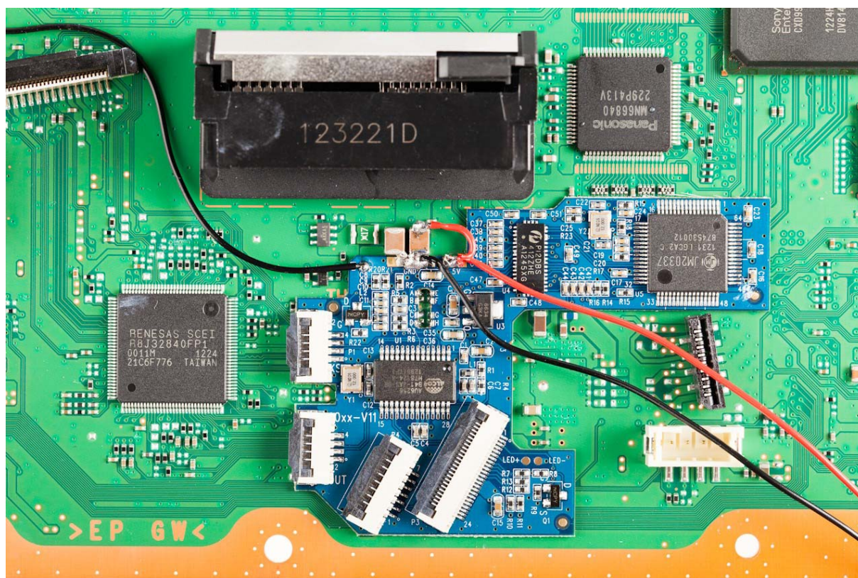
Illustration 6: Montage une fois toutes les soudures terminées
