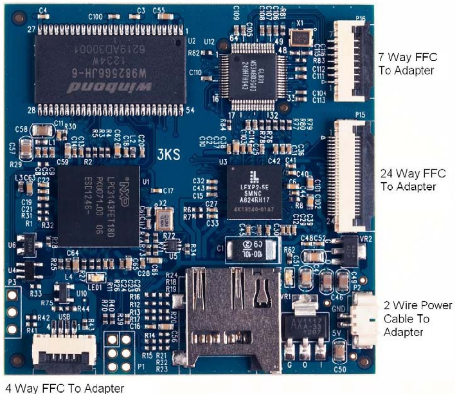
Illustration 12: 3K3y Connecteurs
