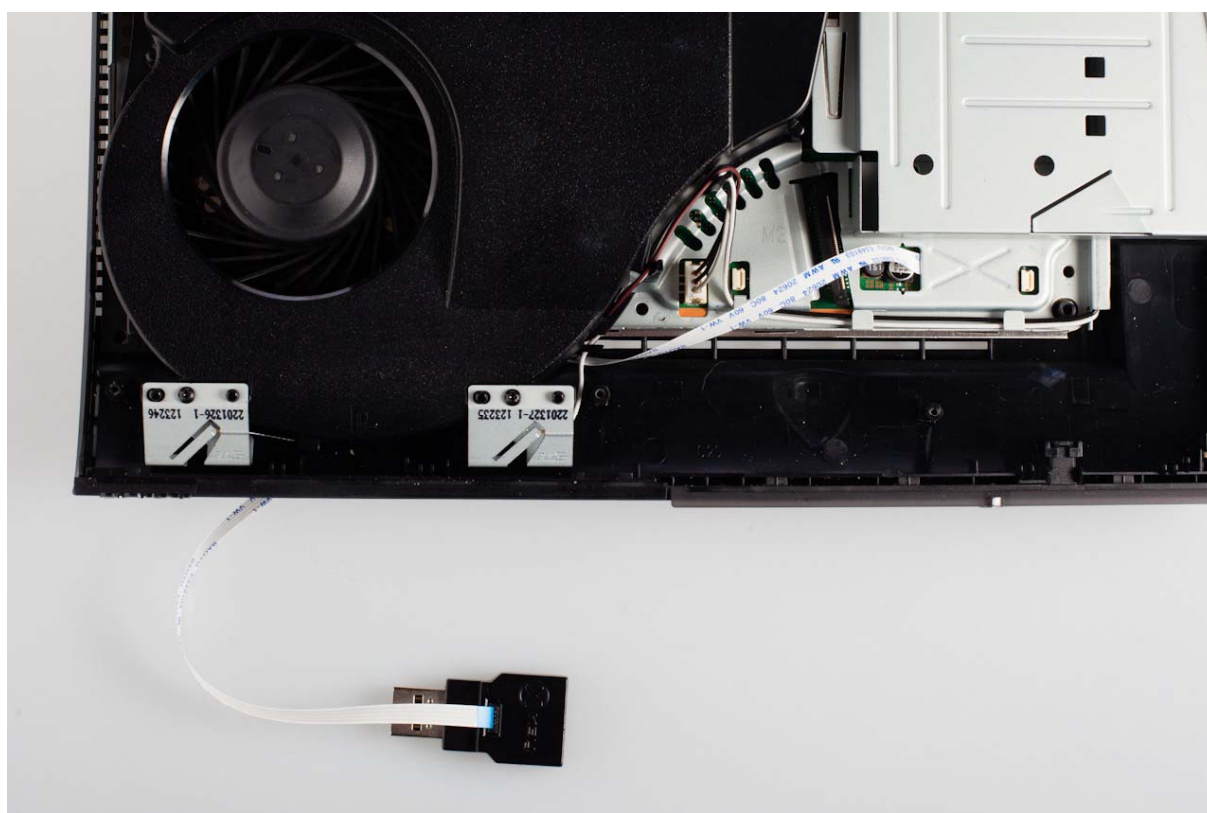
Illustration 15: Mise en place de l'adaptateur USB
