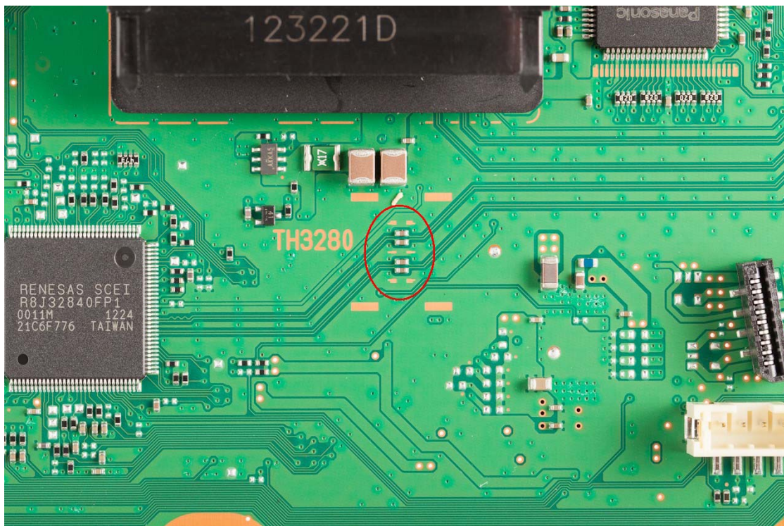
Illustration 2: Gros plan sur les 4 condensateurs du bus SATA
