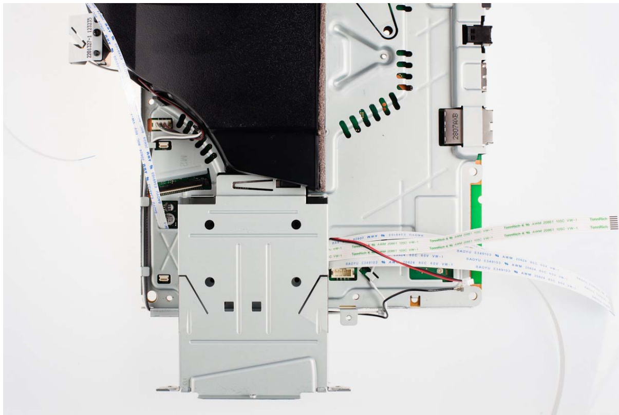
Illustration 9: Remontage du HSF et du blindage
