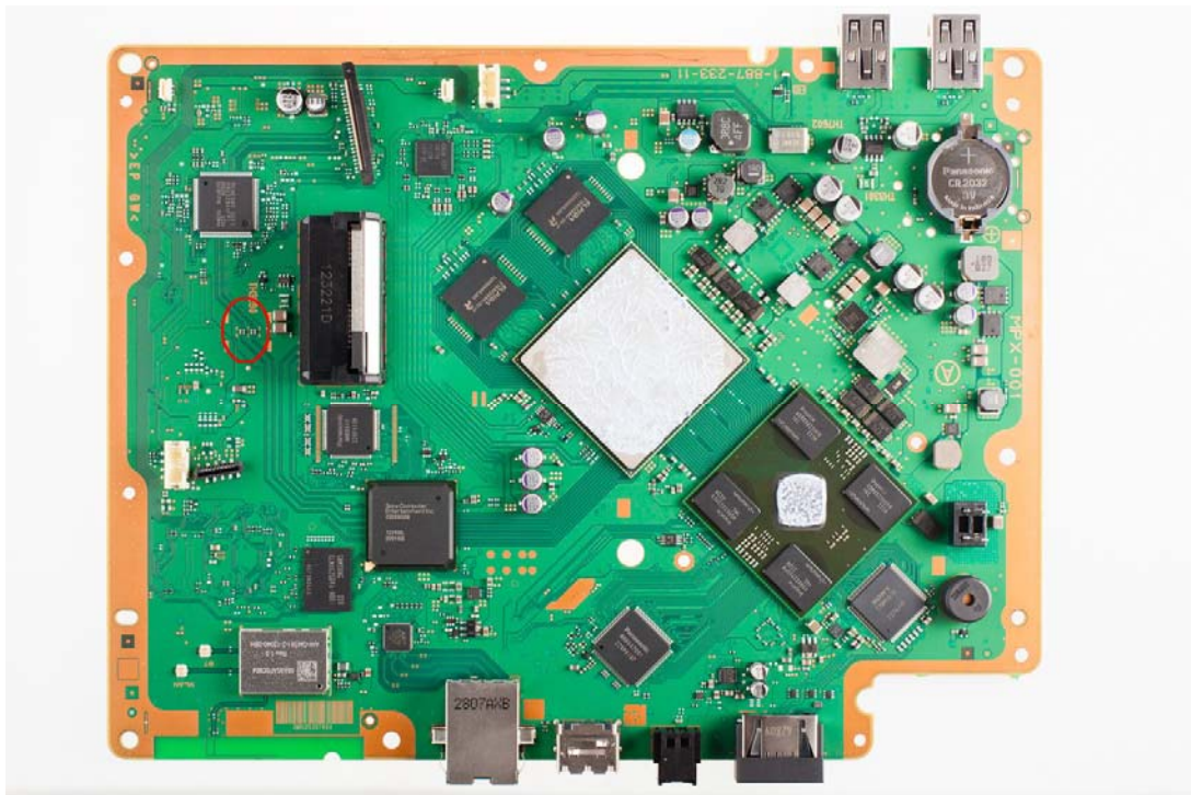
Illustration 1 : Localiser les 4 condensateurs du bus SATA
